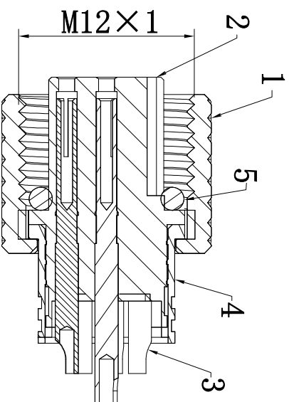
截面 A-A
